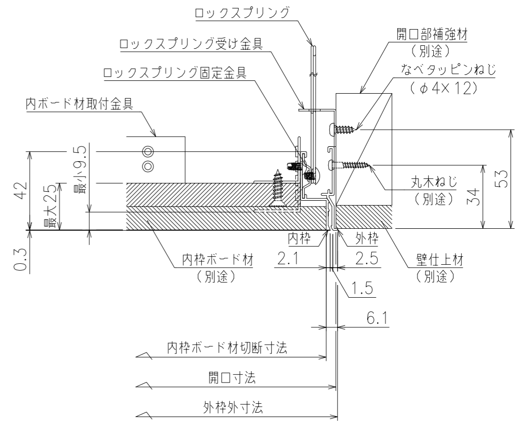
断面納まり図 1:2
